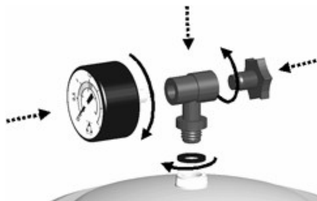
MONTAGE DES MANOMETERS (BEI SEITEN-VENTIL)
